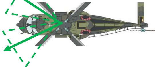
Elicottero con carrello d'atterraggio: Disposizione della fune sul luogo di atterraggio e decollo (raffigurazione simbolica di un NH90, dal web, senza diritti d'autore)
